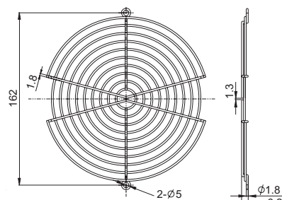
FG-17B For 172mm Fan
