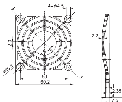
PB-06 For 60mm Fan
